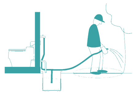
Funktionsschema Ejektortank
